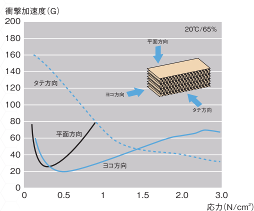
■応力-衝撃加速度線図
