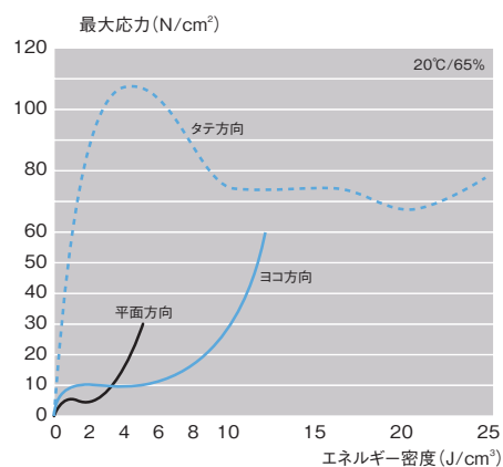
■エネルギー密度-最大応力線図
