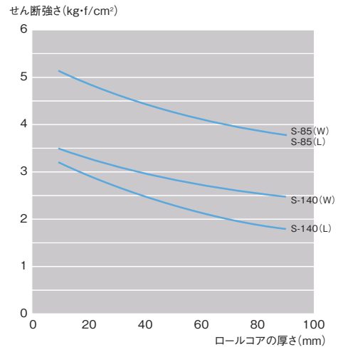
■厚さに対するせん断強さ
