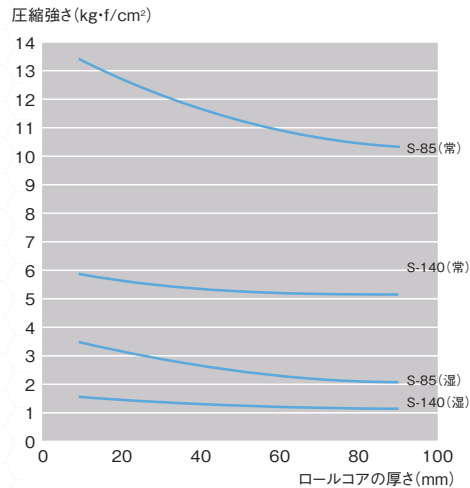
■厚さに対する常態・湿潤圧縮強さ
